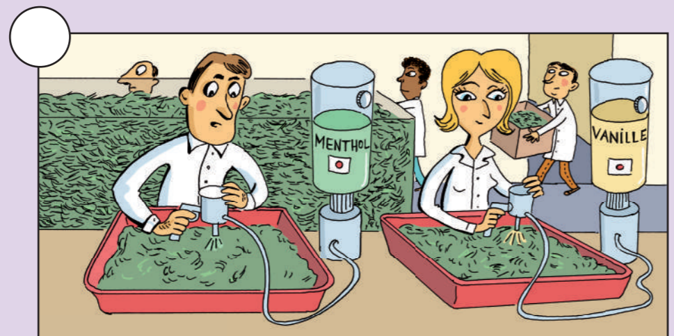
D - Aromatisation
